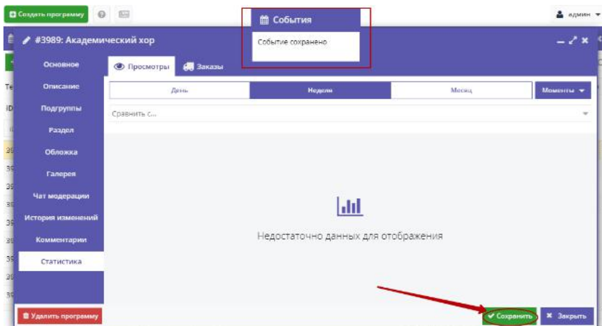
Рисунок 41 – Сохранение Программы
