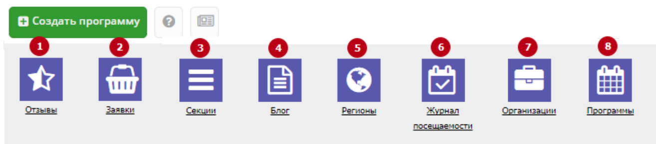
Рисунок 3 – Кнопки инструментов
